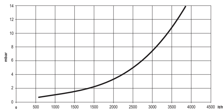
рис. 17 - Гидравлическое сопротивление системы
